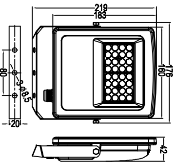
ZY-2085-30W 3030 32颗 16合1
