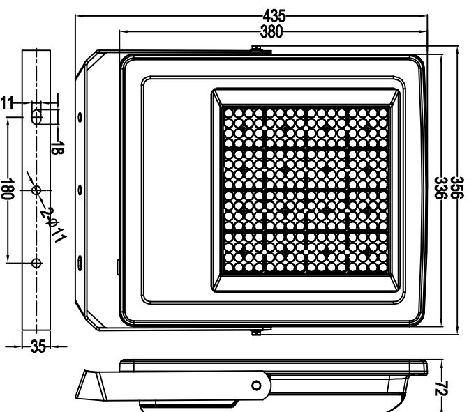
ZY-2085-200W 3030 256颗 16合1
