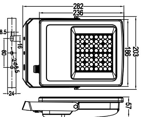
ZY-2085-50W 3030 64颗 16合1
