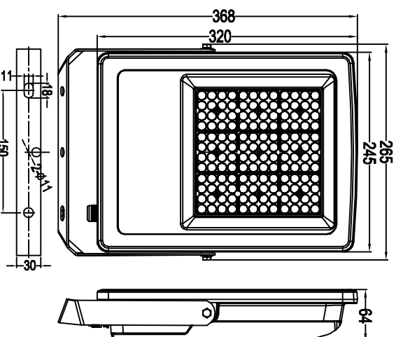
ZY-2085-100W 3030 144颗 16合1
